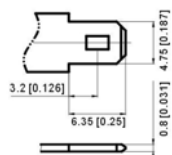
Клемма F1
