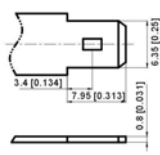
Клемма F2
